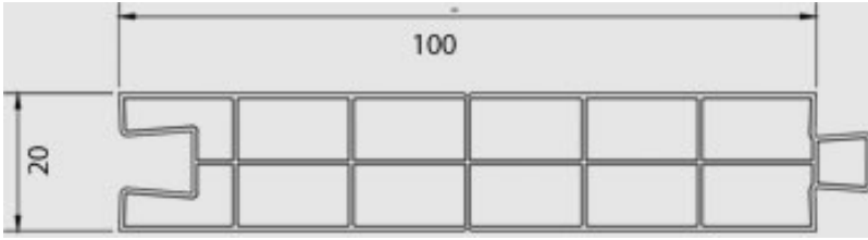
Teknik Çizim
